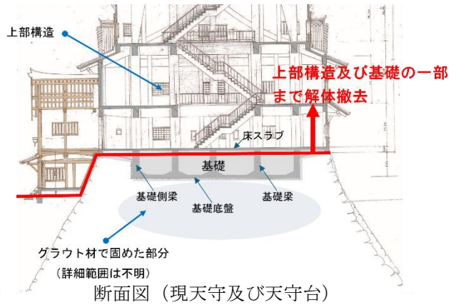
断面図（現天守及び天守台）
